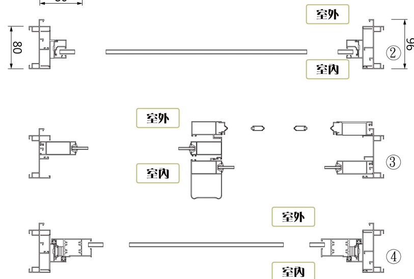
◄ 橫向剖面圖
