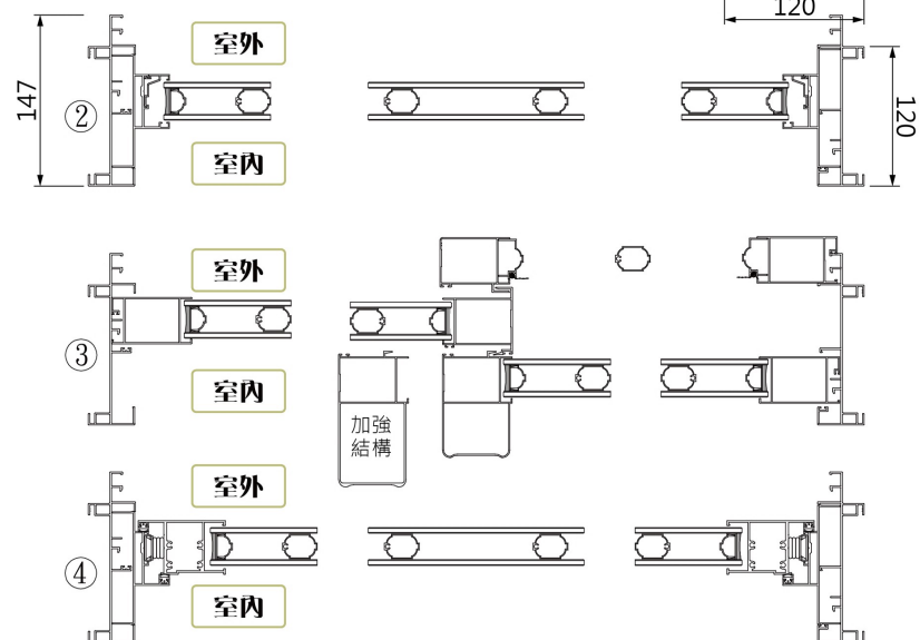
► 橫向剖面圖
