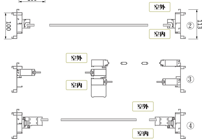
▶ 橫向剖面圖
