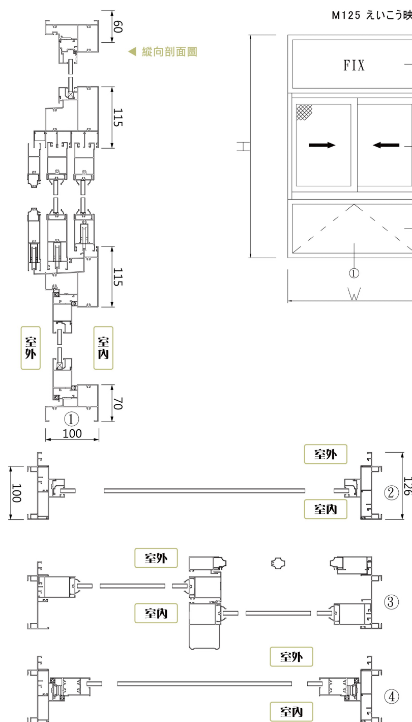
▶ 橫向剖面圖
