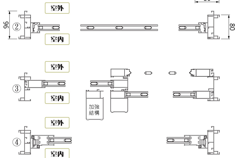
► 橫向剖面圖
