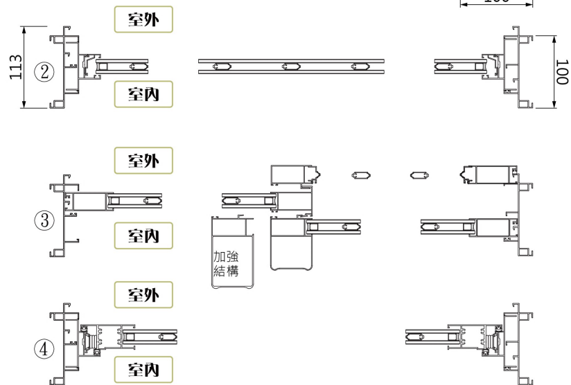
▶ 橫向剖面圖
