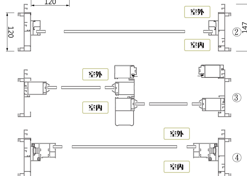
► 橫向剖面圖
