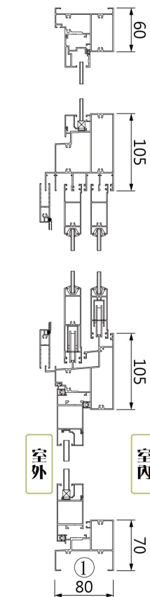
◄ 縱向剖面圖
