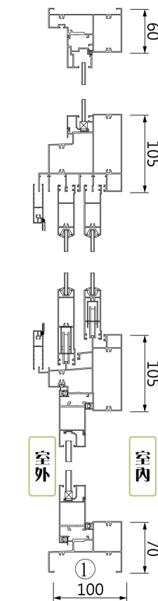
▶ 縱向剖面圖
