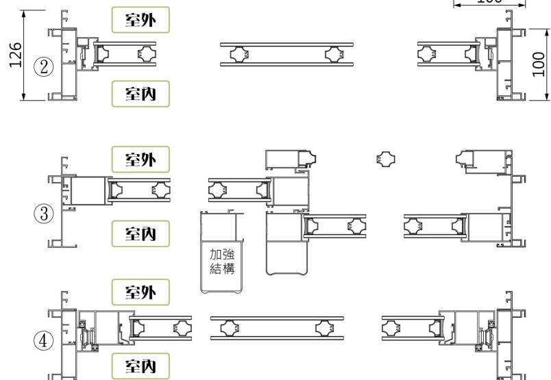
▶ 橫向剖面圖
