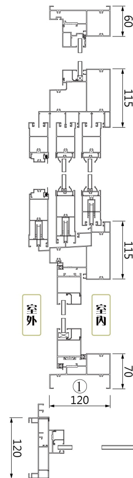
► 縱向剖面圖
